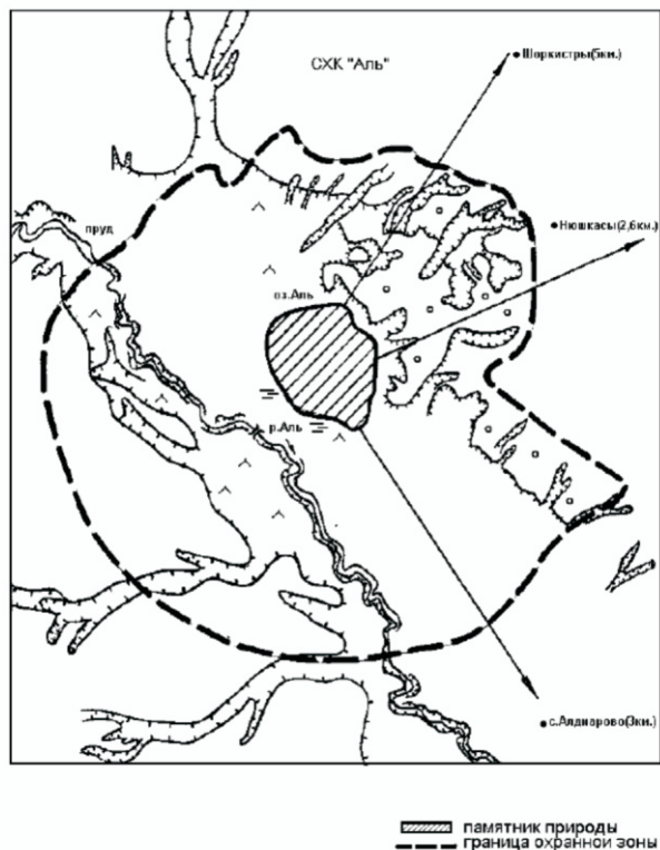
Схема расположения памятника природы «Озеро Аль». Масштаб 1:10000
